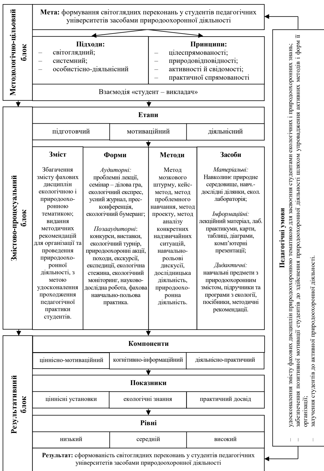
Рис. 1. Модель формування світоглядних переконань у студентів педагогічних університетів засобами природоохоронної діяльності
