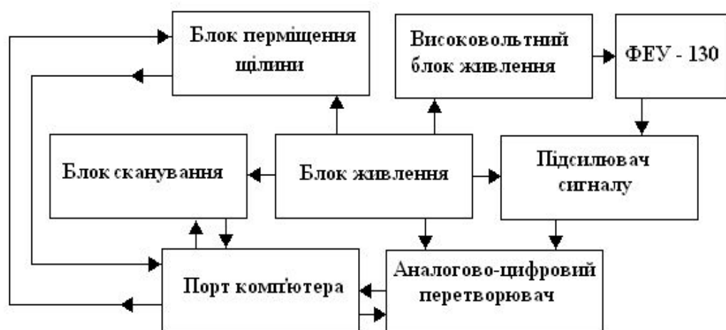
Рис. 2. Структурна схема електричної частини приладу
